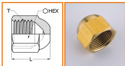
螺帽蓋 Cap Nut
