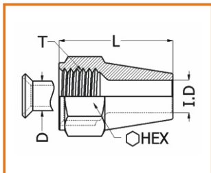
長螺帽 Long Nut
